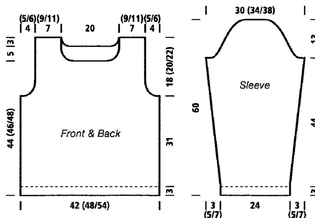
Etu- ja takakappale
