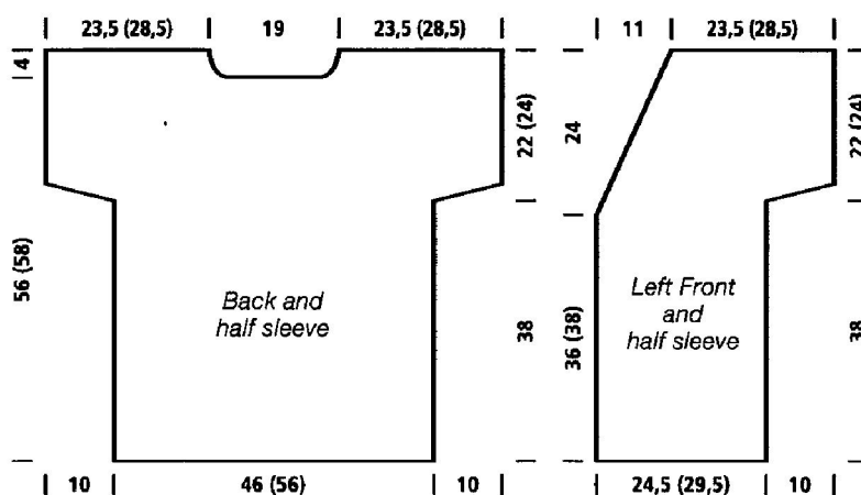
Takakappale ja puolet hihoista
